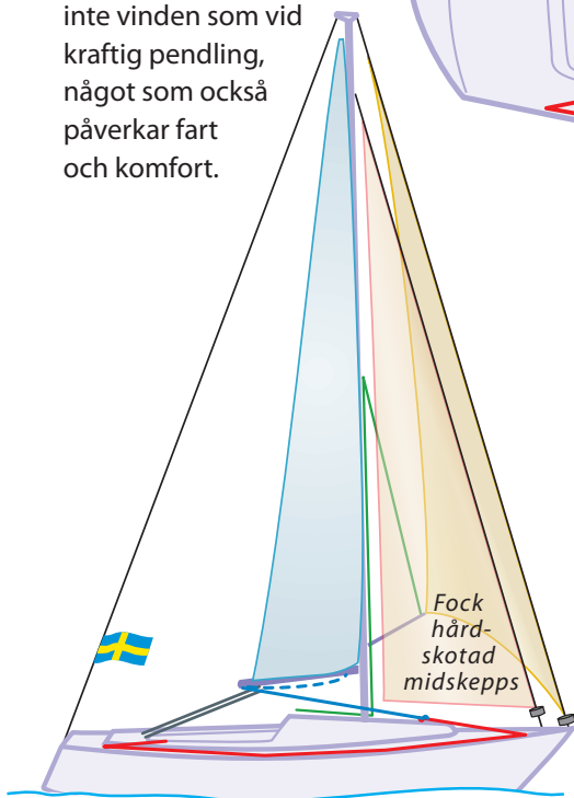
Principskisser. Illustrationerna är ej skalriktiga.
